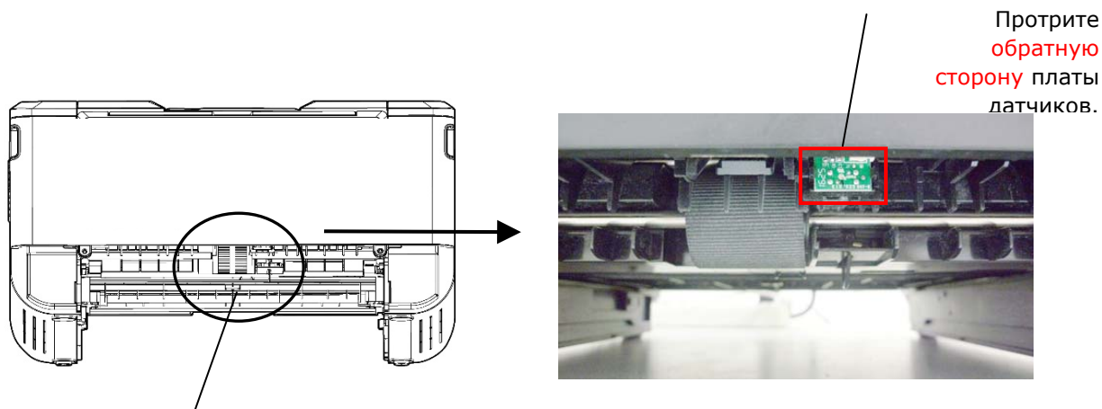
Ролик захвата бумаги
