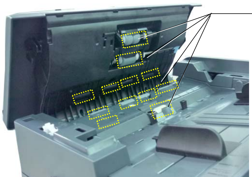
Подающий ролик
